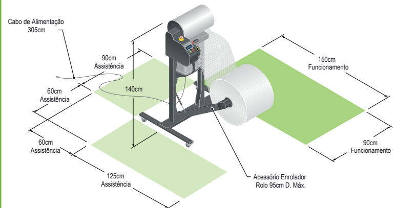
Configuração do Sistema - Suporte com Versão de Enrolador de Rolo
